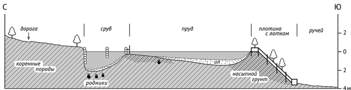
Рис. 4. Схематический профиль Поповского пруда
