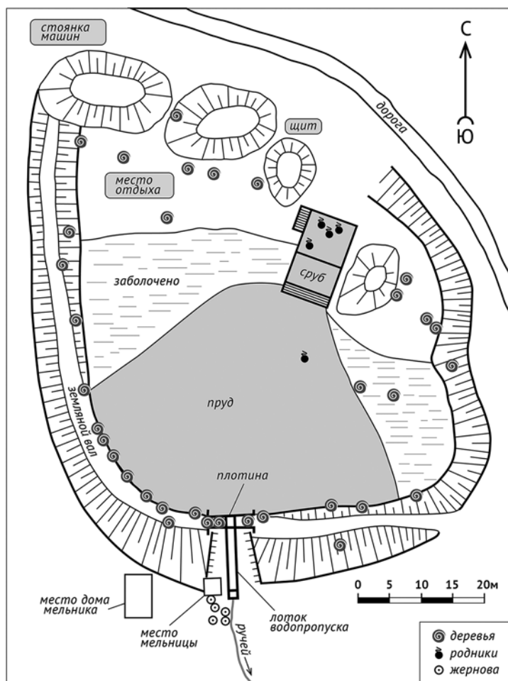
Рис. 2. Схема родникового пруда (обмеры 2019 г., тахеометрическая основа А. Н. Филина)
